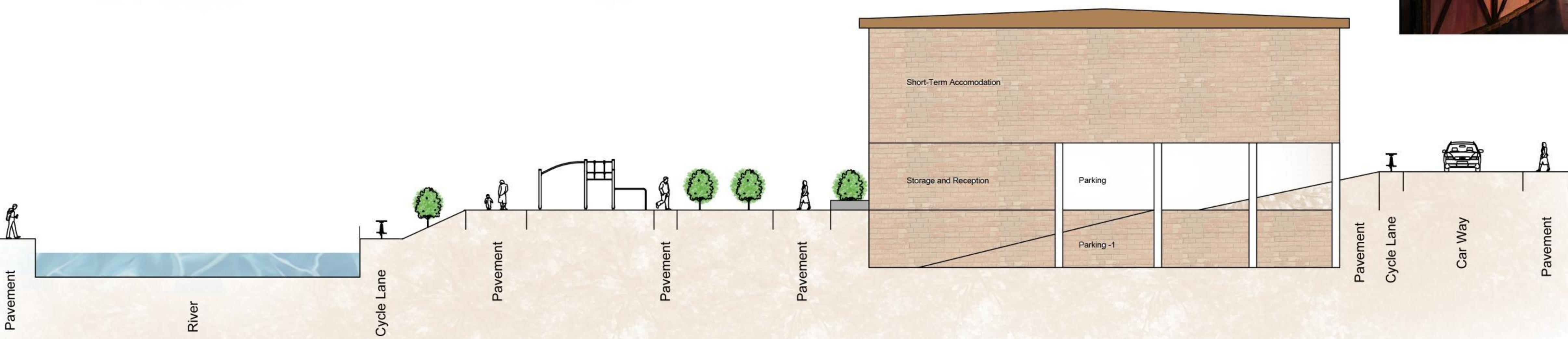
Section A-A Scale: 1/200
